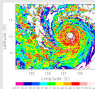
フィリピンで大災害を与えた2013年台風30号(ハイエン)の再現計算から作成した疑似レーダー降水画像 Radar precipitation from a computer simulation of Typhoon Haiyan (2013) which caused heavy disaster in Philippines
