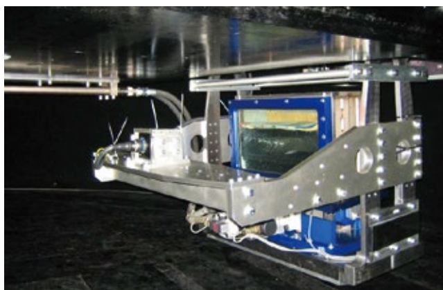
土槽搭載時の遠心力装置 Geotechnical centrifuge at DPRI
